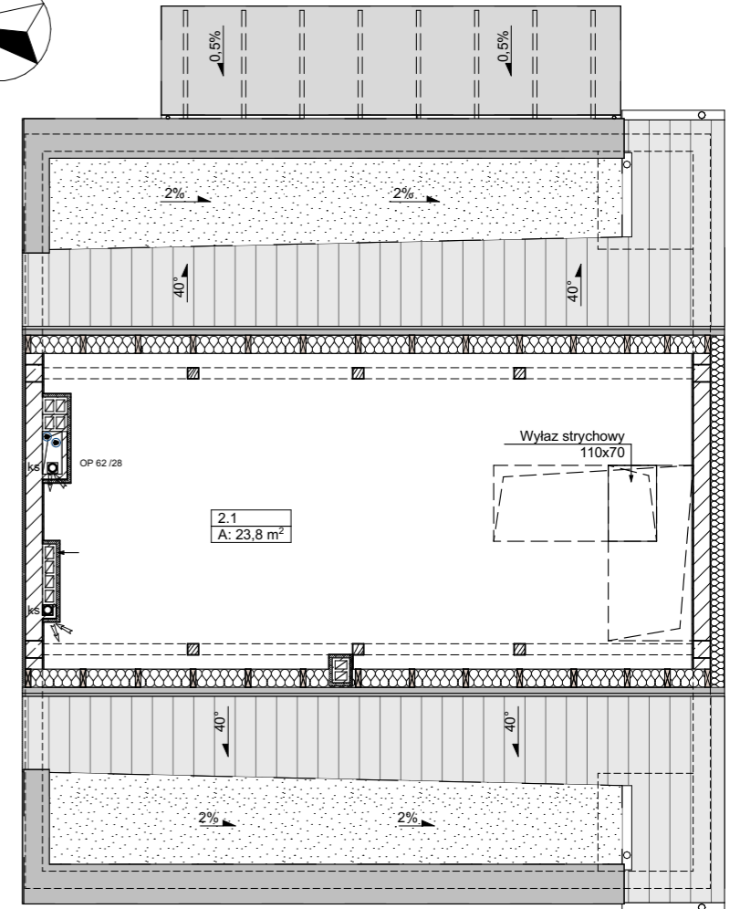
Rzut antresoli +2
