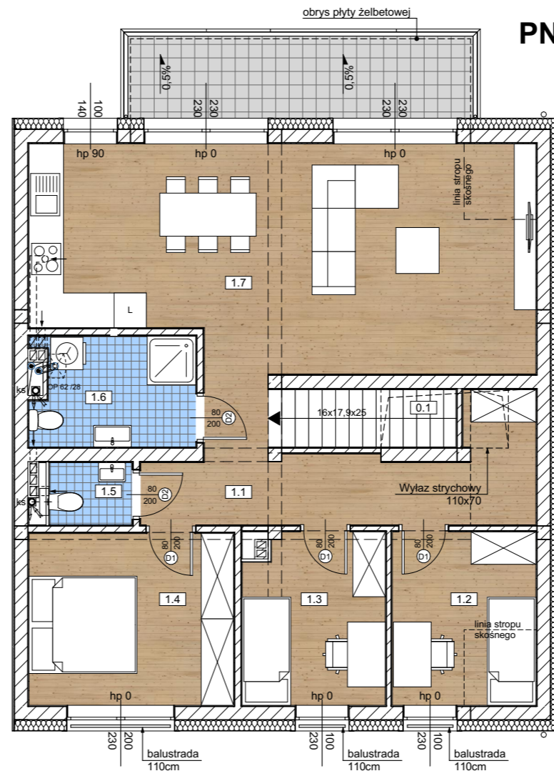
Rzut piętara +1
