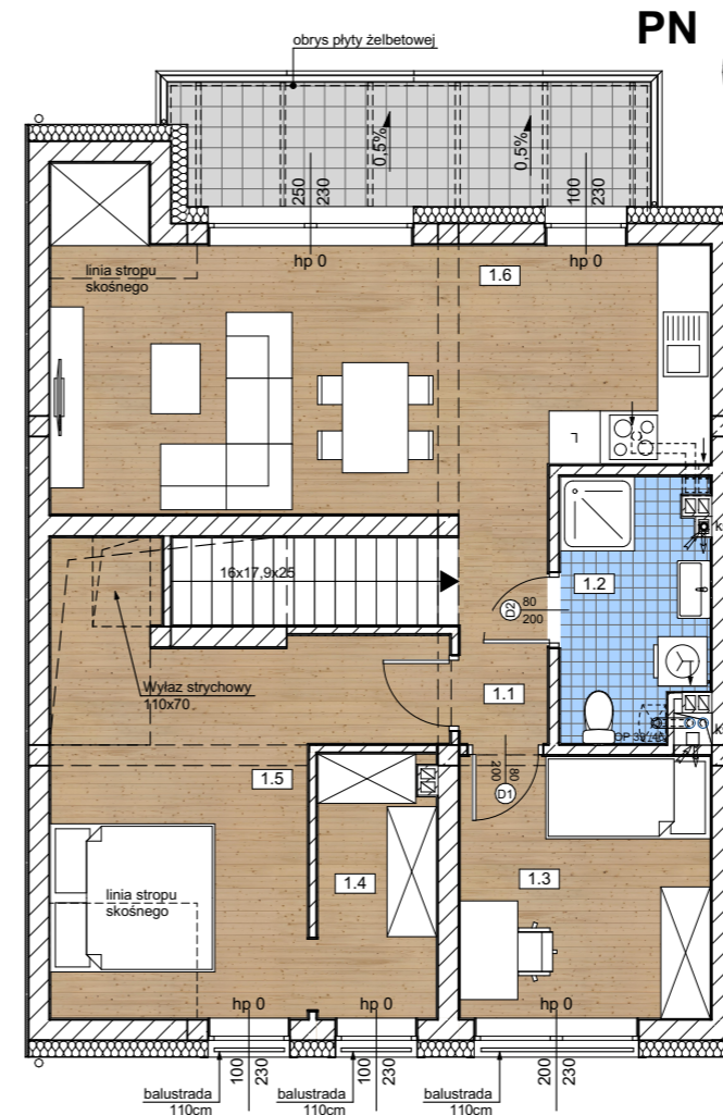
Rzut piętra +1
