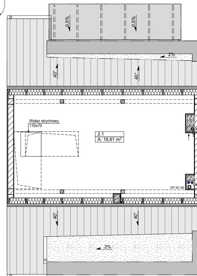
Strych +2
