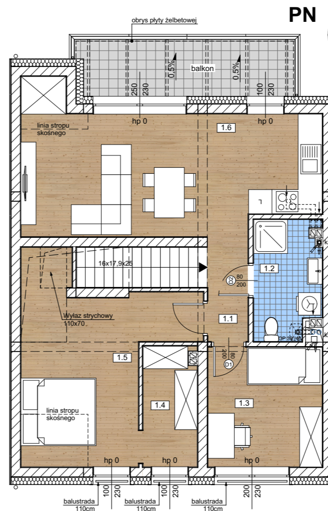
Rzut piętra +1
