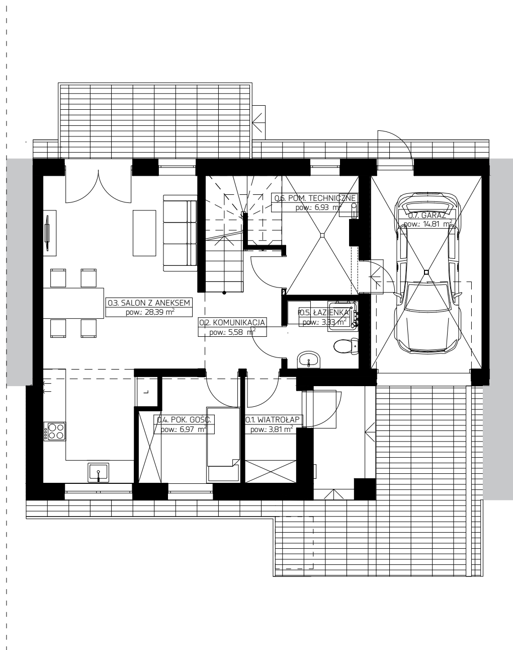
BUDYNEK MIESZKALNY W ZABUDOWIE SZEREGOWEJ PARTER
