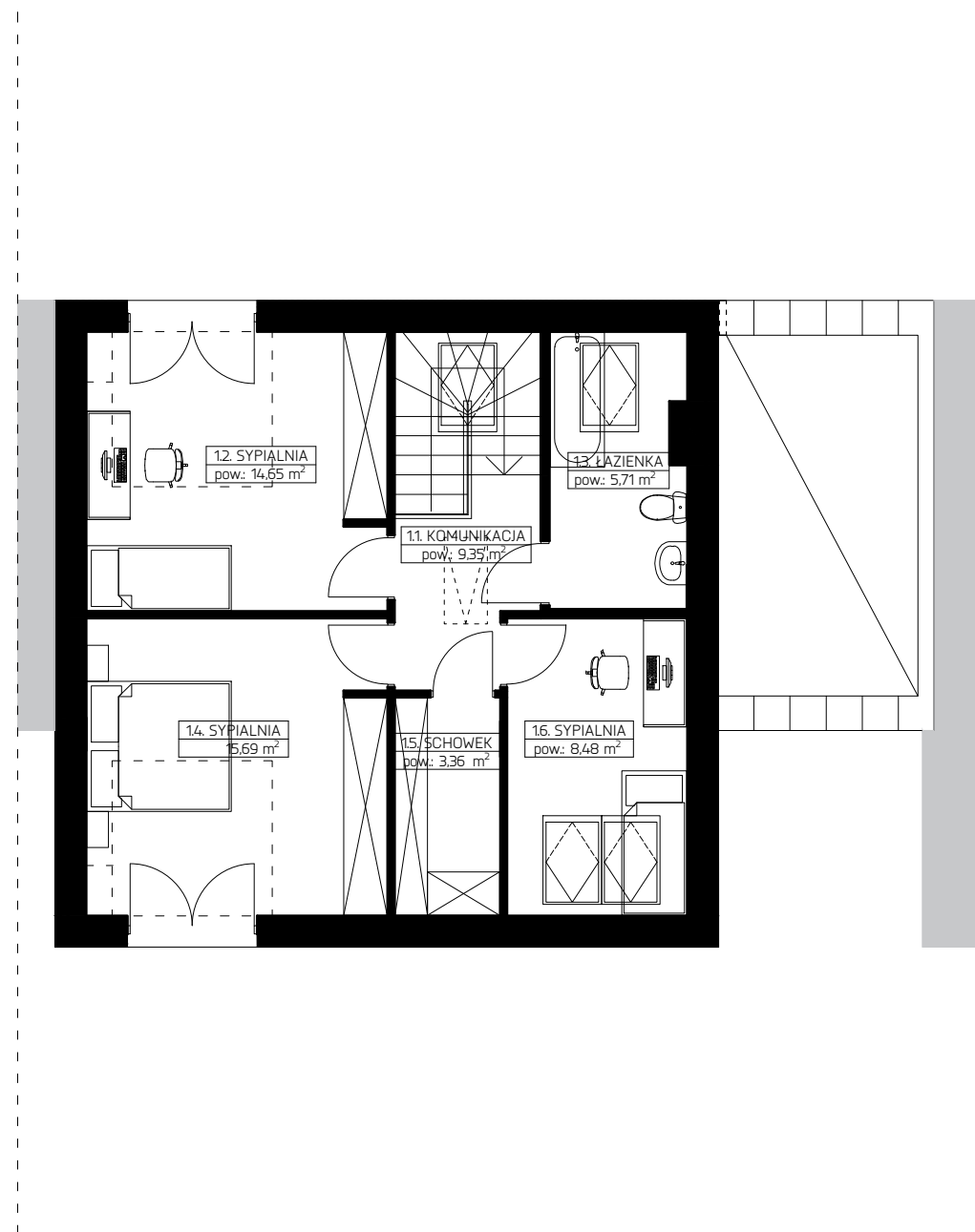
BUDYNEK MIESZKALNY W ZABUDOWIE SZEREGOWEJ PIĘTRO
